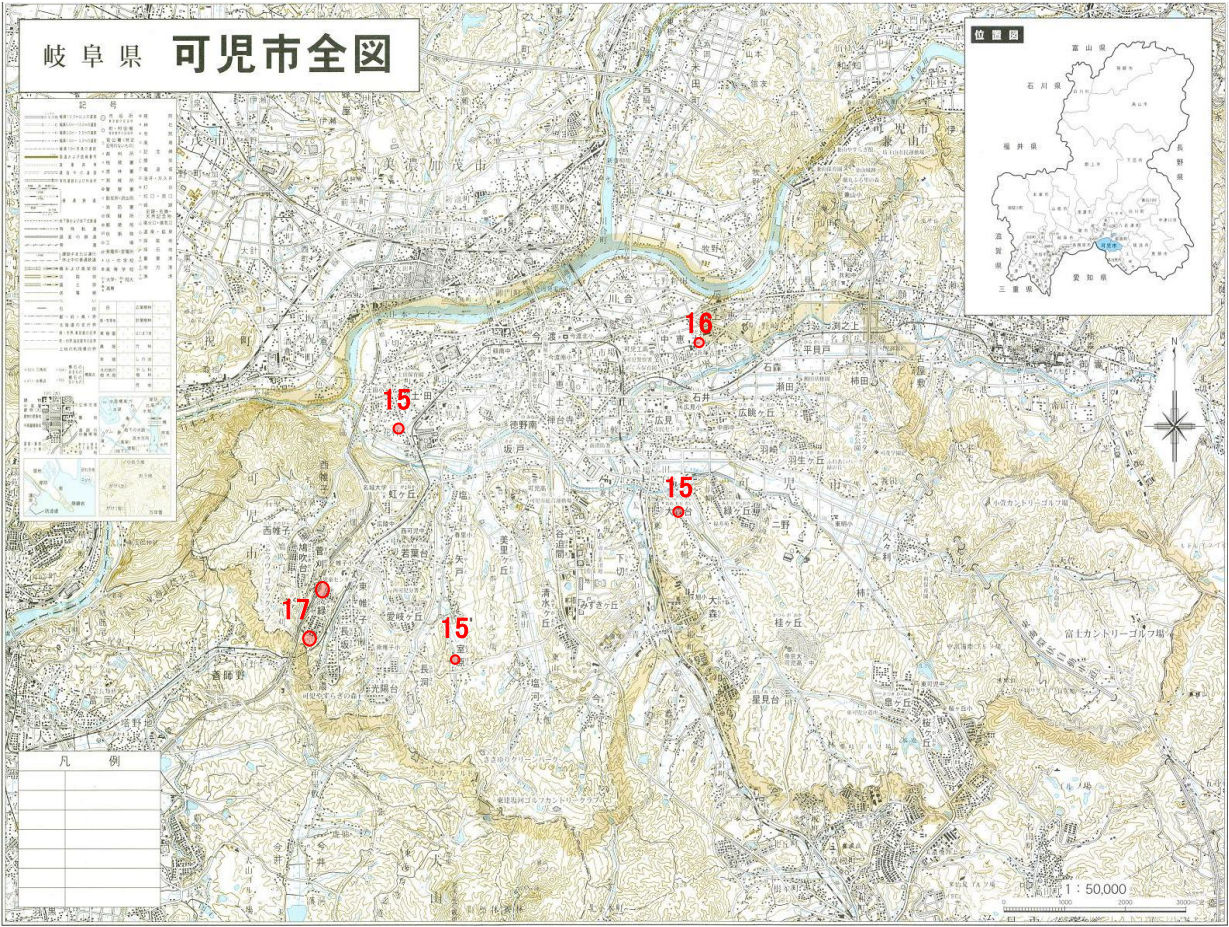
施工位置図
