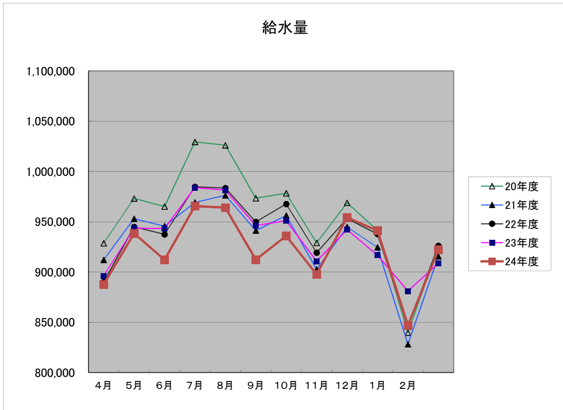
給水量 (m 3 )
