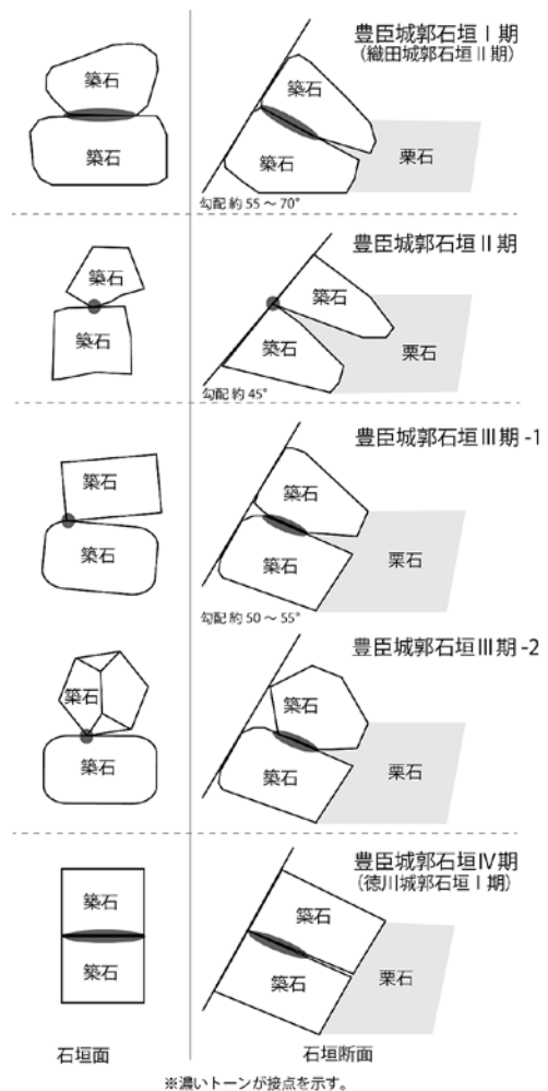
図65 豊臣城郭石垣の築石接点変遷モデル（下高2017）
