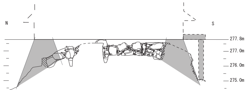
図77 石垣復元図（西より）
