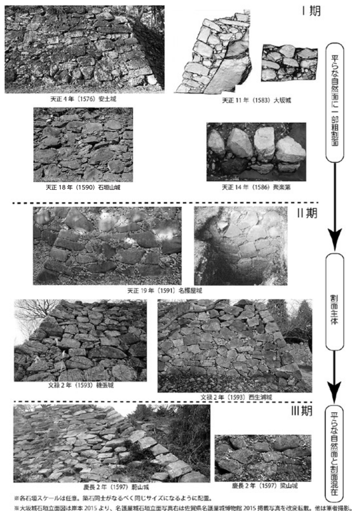
図64 豊臣城郭石垣の石垣面変遷（下高2017）
