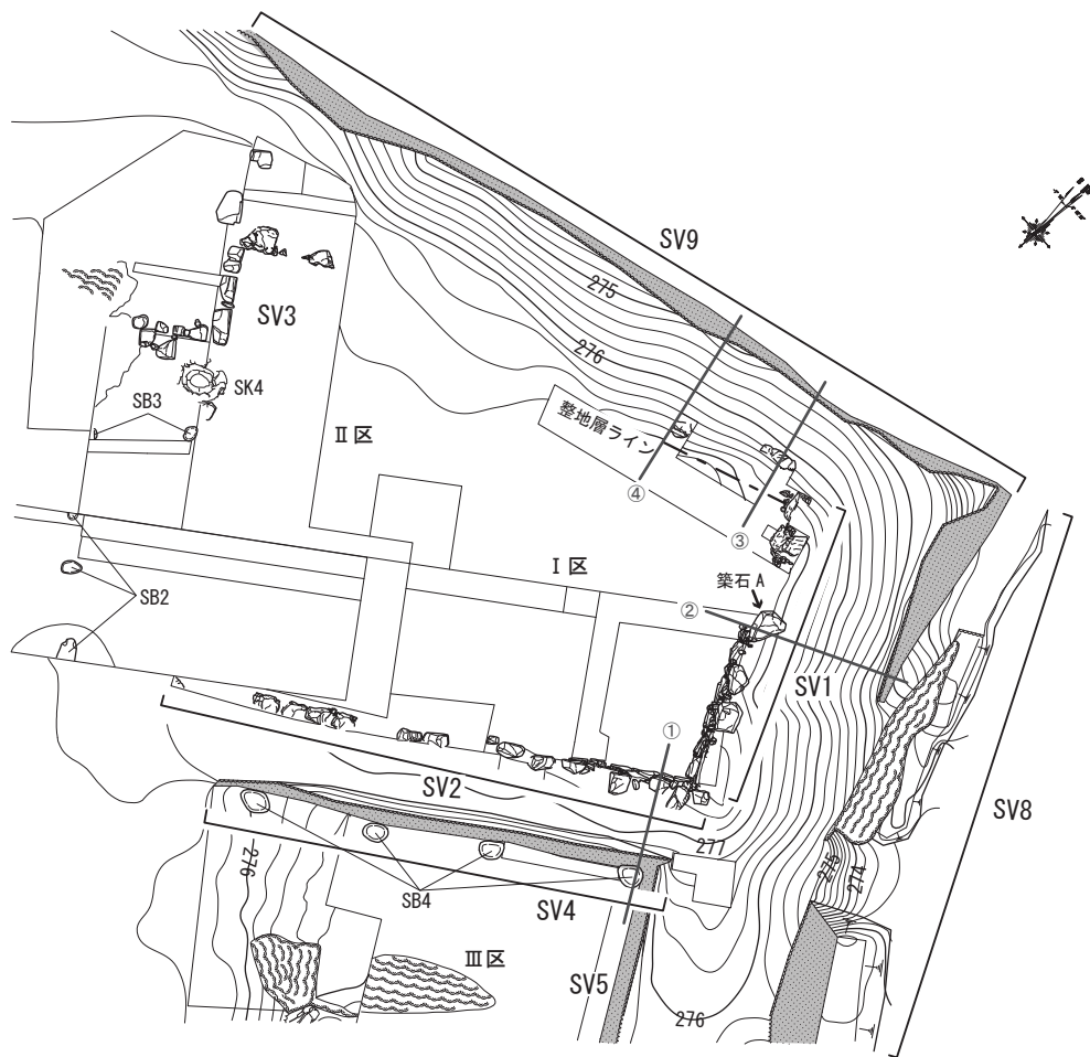
図67 断面位置図(第2期の遺構)
