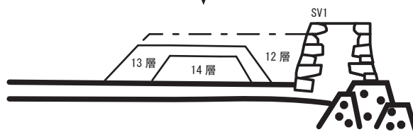
③12 層が入れられた段階
