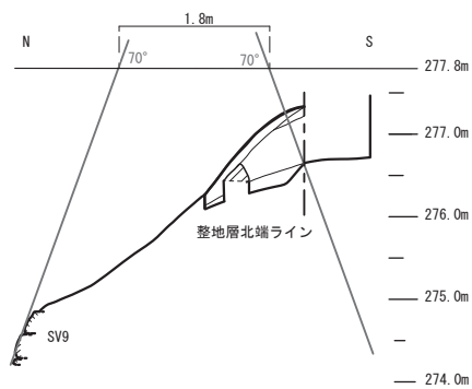
図71 石垣断面④復元図
