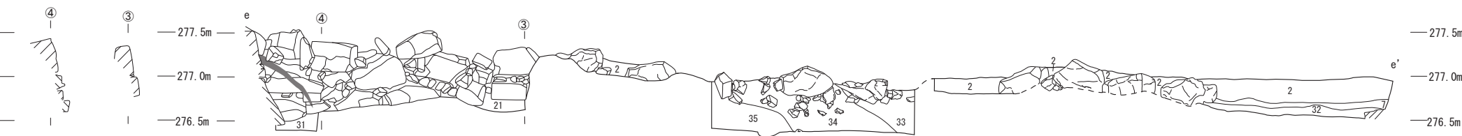
図 10 SV2 立面図及び e-e' 土層図
