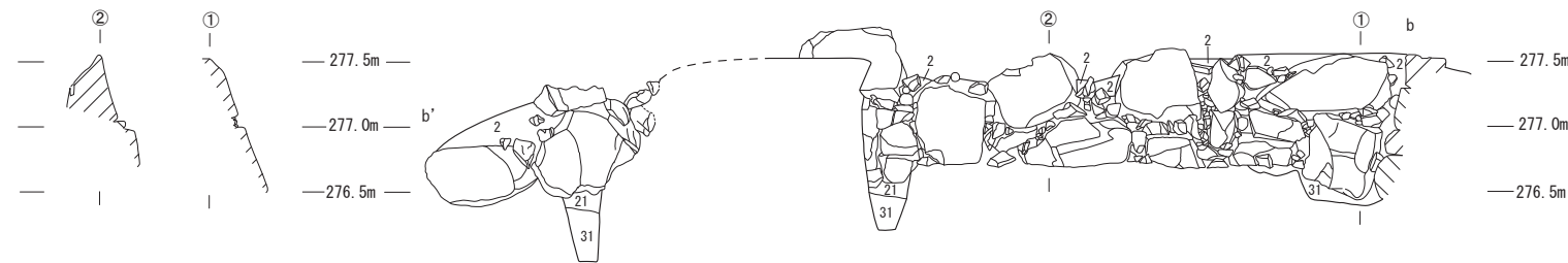
図 7 SV1 立面図及び b-b' 土層図
