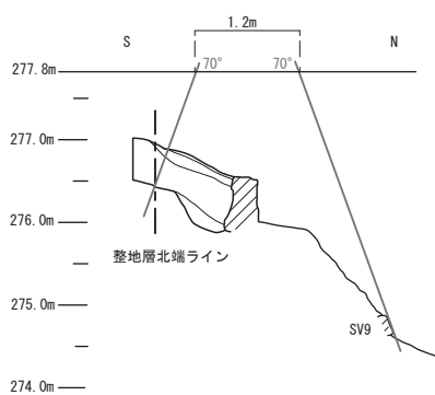
図70 石垣断面③復元図
