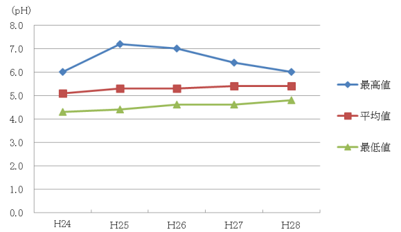
降雨中のpHの推移
