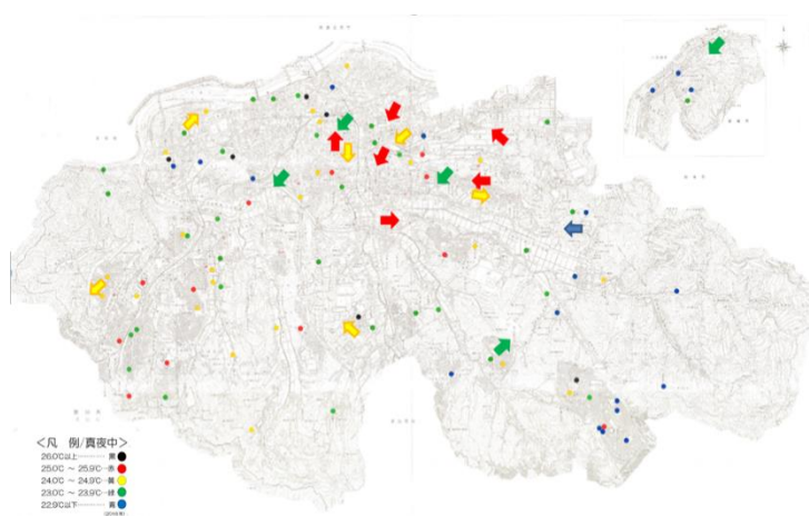
観測気温分布図（平成 28 年 8 月 1 日真昼）
