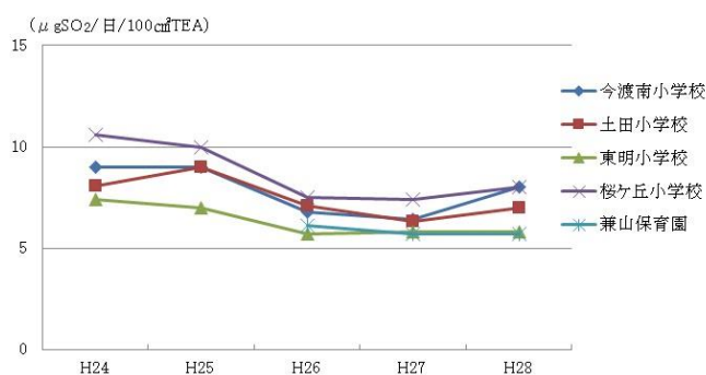
二酸化硫黄 (SO 2 ) の推移
