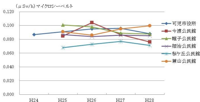
空間放射線量の推移
