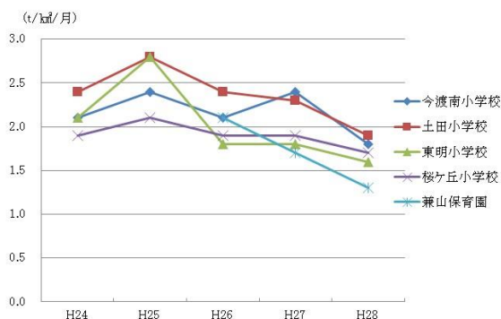
降下ばいじんの推移
