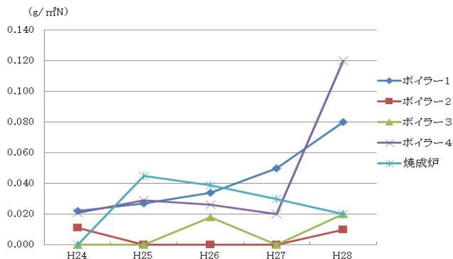
ばいじん濃度の推移
