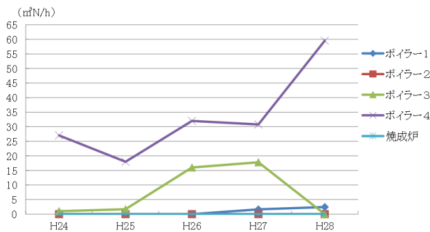
ばいじん濃度の推移
