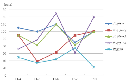
窒素酸化物の推移
