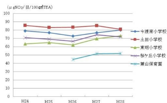
二酸化窒素 (NO 2 ) の推移
