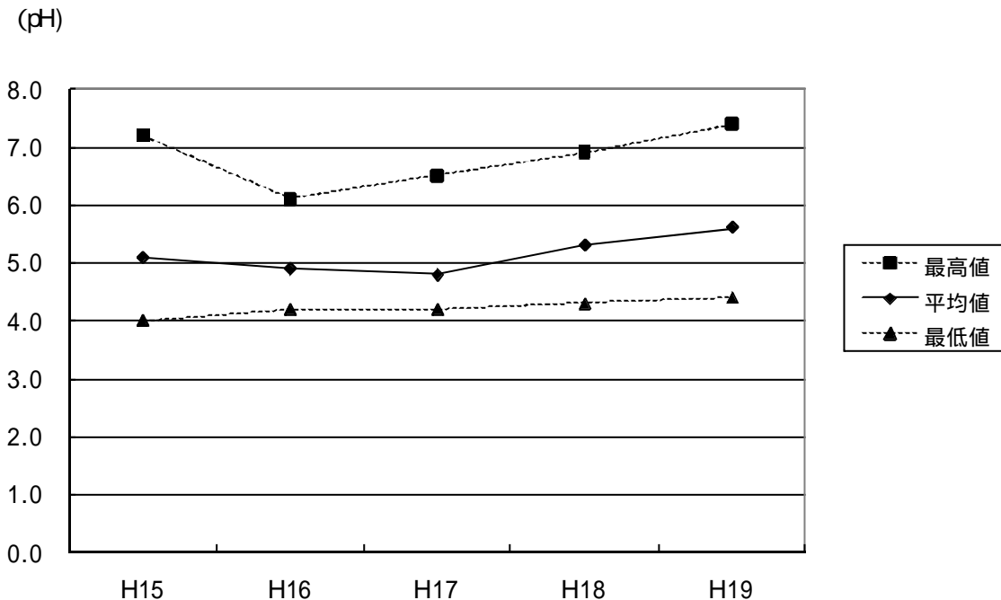
図 -1-4 降雨の pH 測定値経年変化 (ろ過式雨水採取装置)
