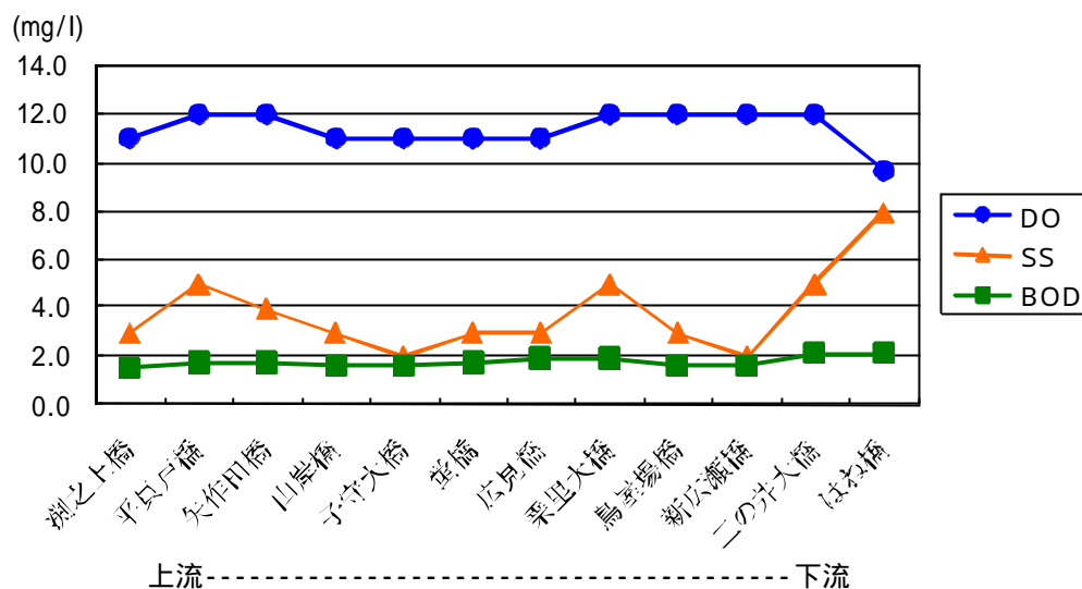
図 -2-1 可児川本川水質流下変化 [年平均値]
