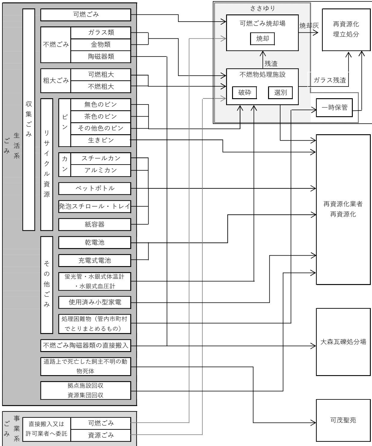
ごみ処理フロー
