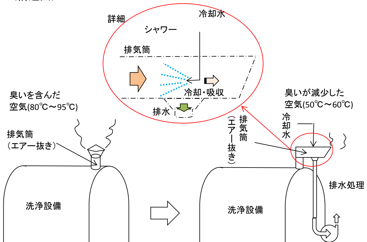
(構造図)
