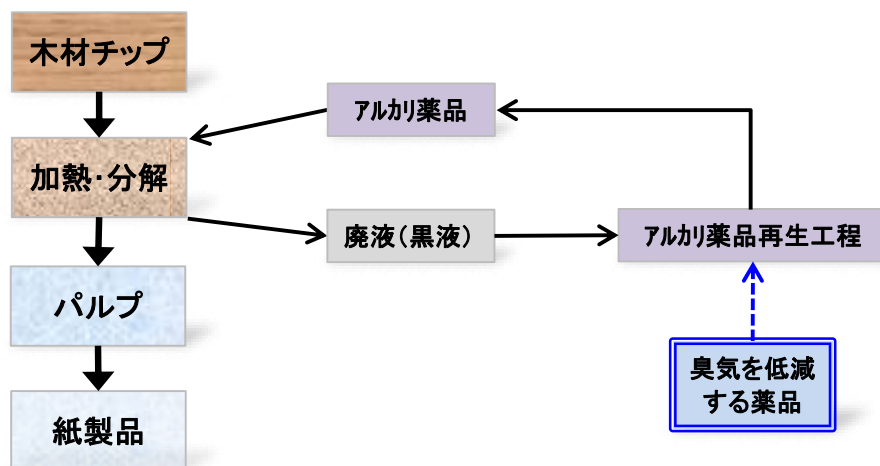
【アルカリ薬品再生フロー】
