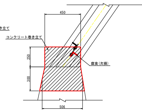
3 - 3 S=1:10
