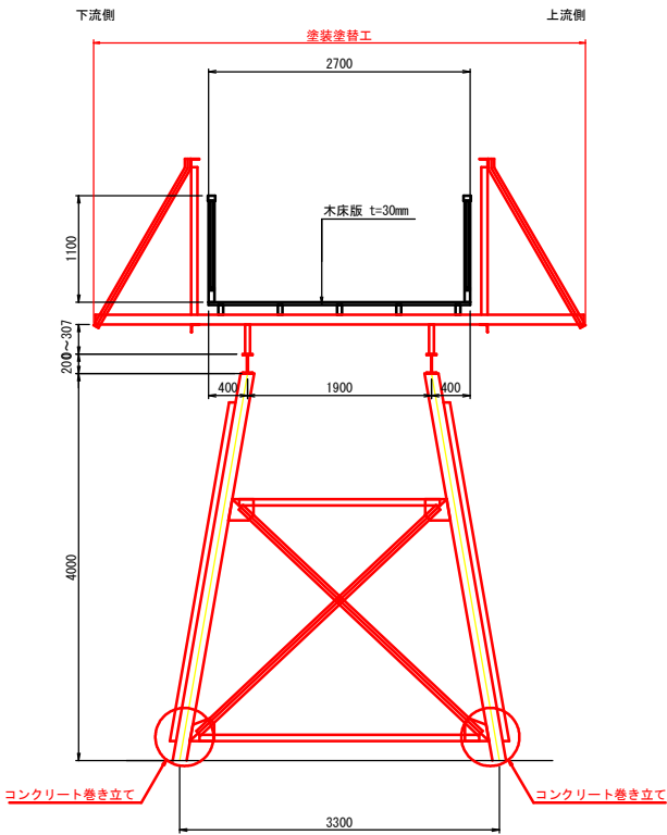
断面図 S=1:30
