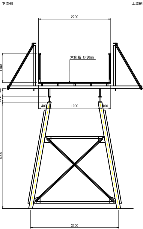
断面図 S=1:30
