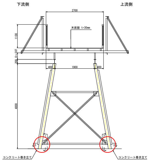
断面图 S=1:50
