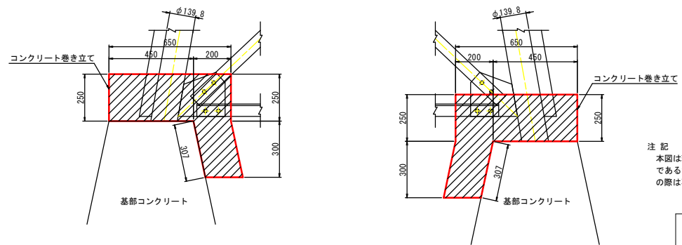
4 - 4 S=1:10
