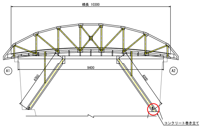
側 面 図 S=1:50
