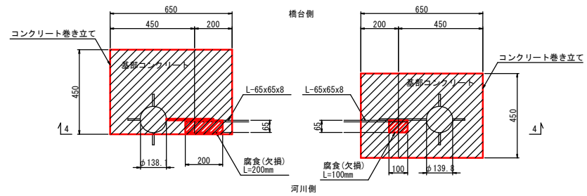
3 - 3 S=1:10
