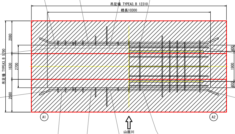
平面図 S=1:50
