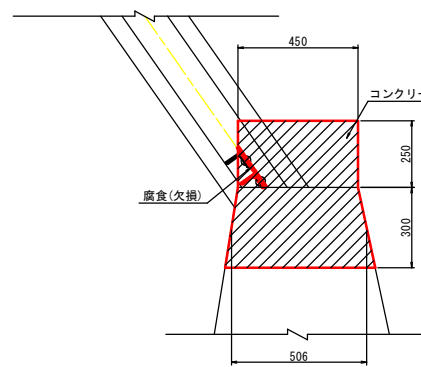
1 - 1 S=1:10
