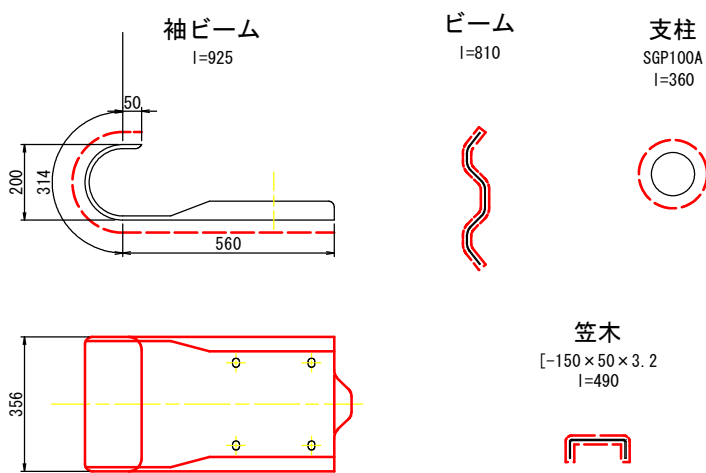
塗装範囲
