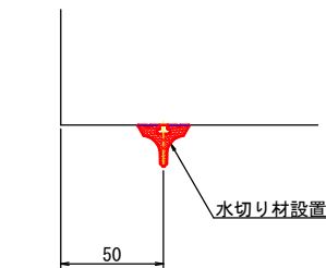
水切り詳細図
