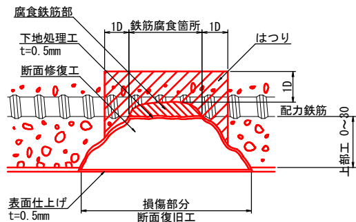
左官工法
