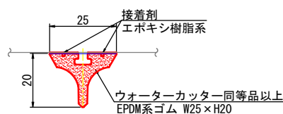
水切り詳細図
