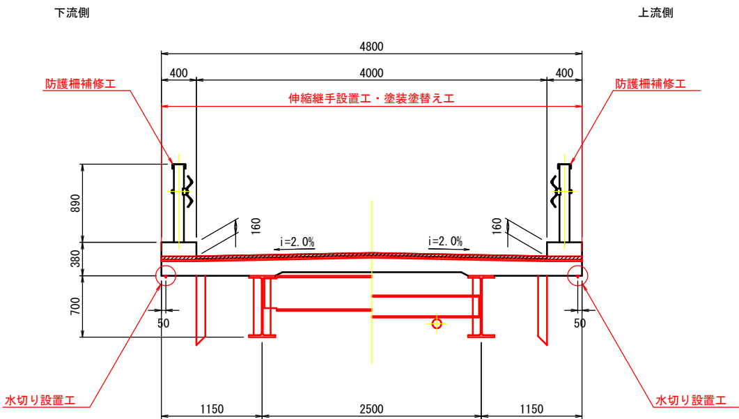
断 面 図
