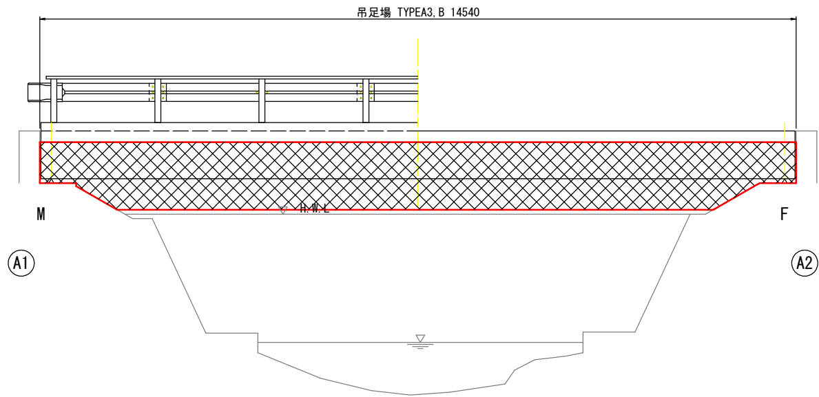
平面図
