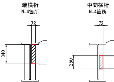
横桁交差部詳細図
