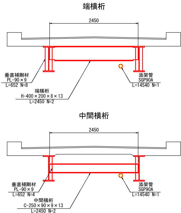
断面図
