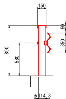
断 面 図
