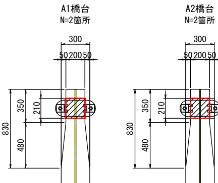
支承交差部詳細図
