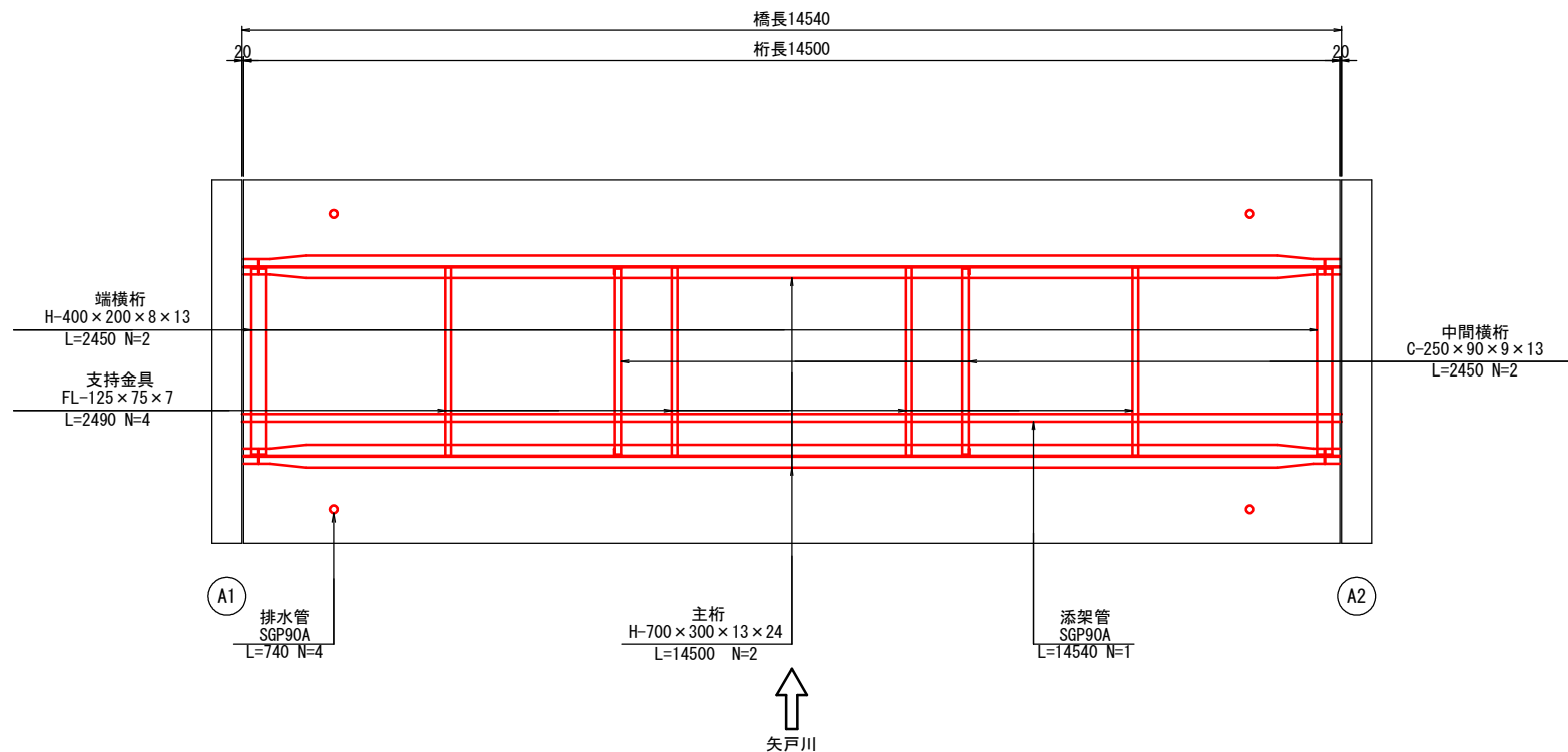
支承
