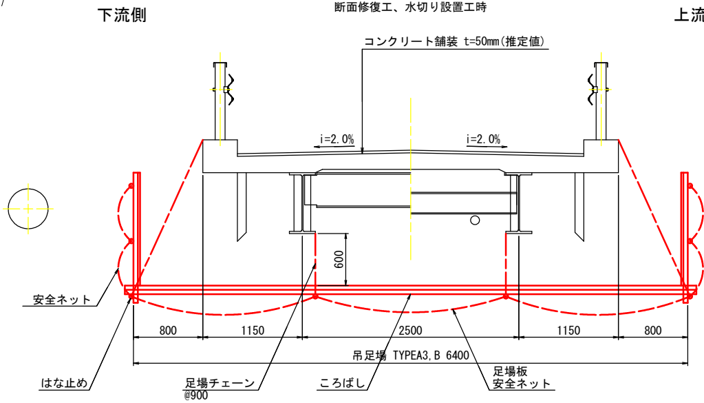
断面図
