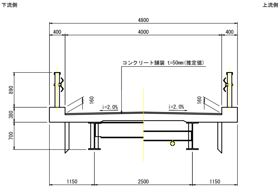
断 面 図
