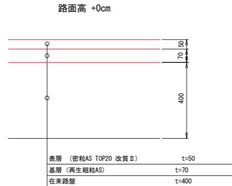
舗装構成 (計画) S=1:10
