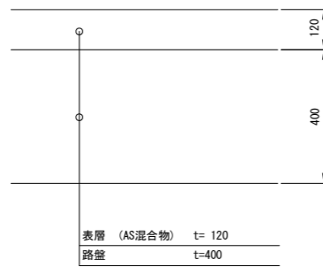
舗装構成 (現況) S=1:10
