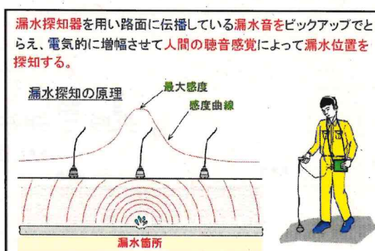
路面音聴調査図
