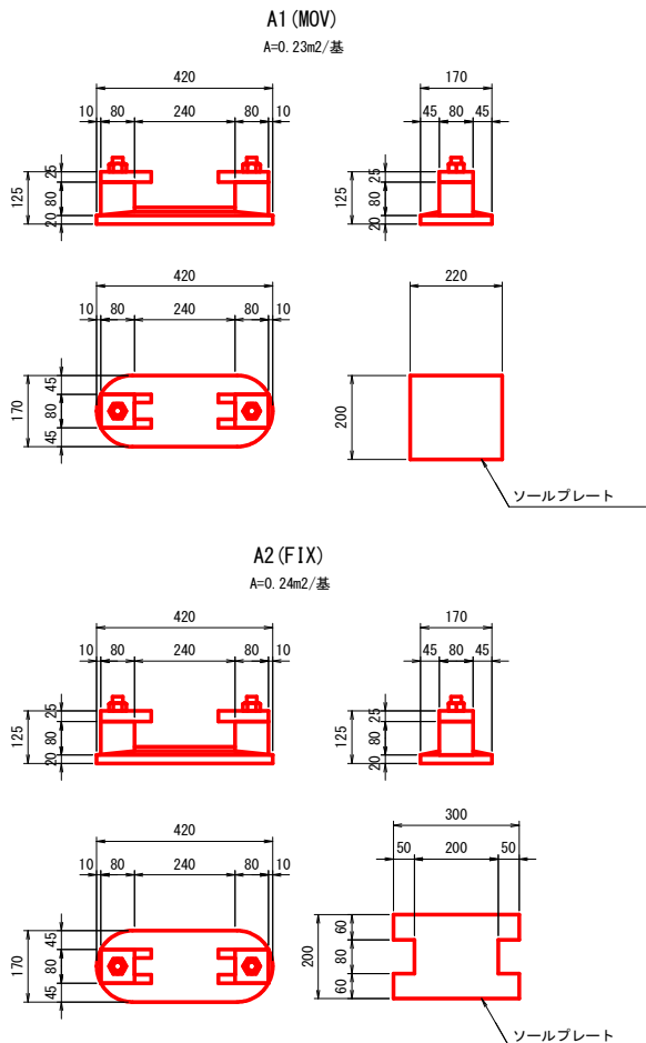
支承 S=1:10
