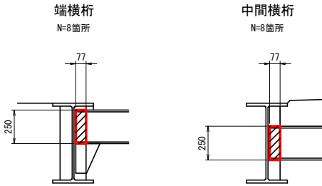
横桁交差部詳細図 S=1:20
