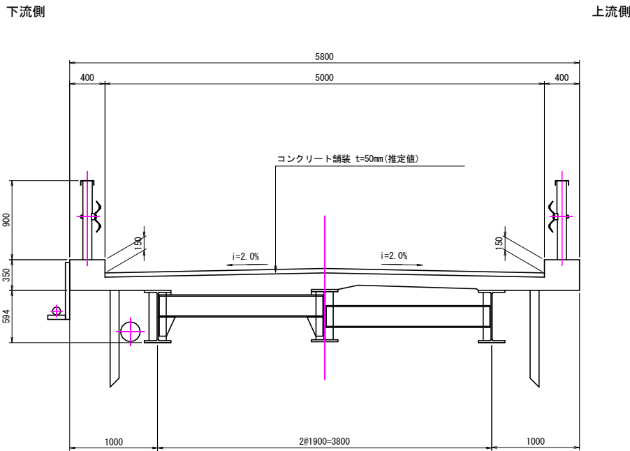
断面図 S=1:30
