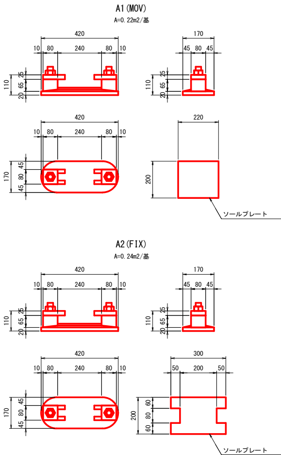
支承 S=1:10
