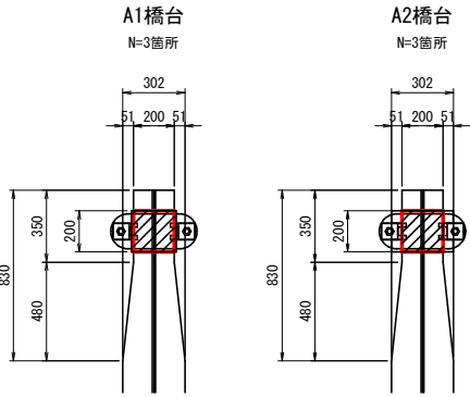
支成交差部詳細図 S=1:20
