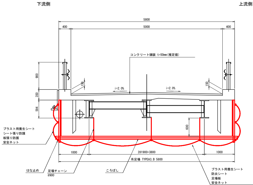
断面図 S=1:30
