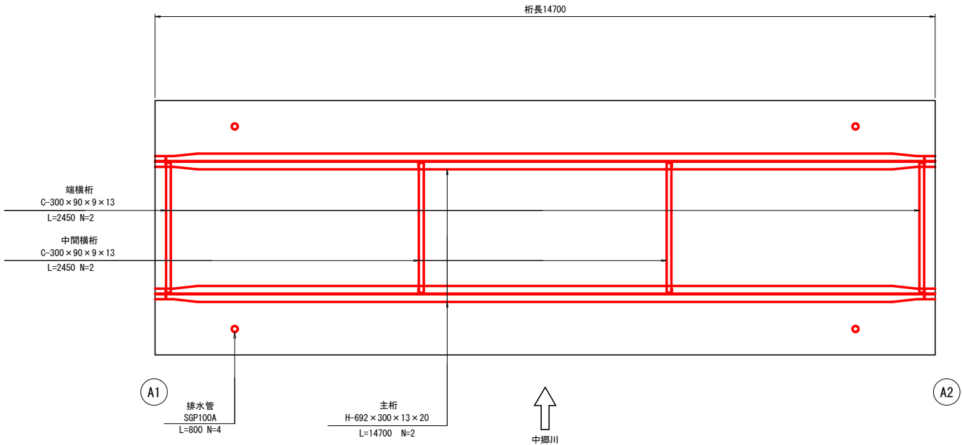
平面図 S=1:50
