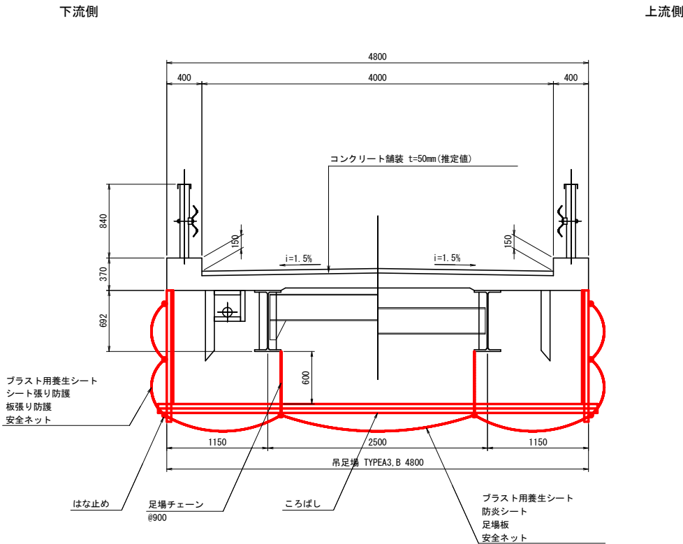
断面図 S=1:30
