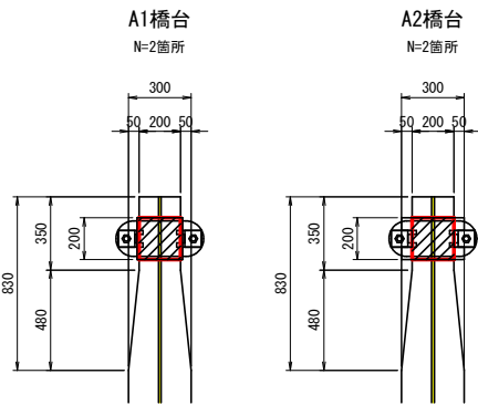
支承交差部詳細図 S=1:20
