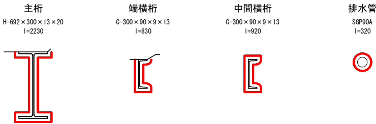
塗装範囲 S=1:20
