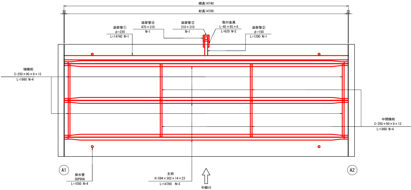
平面図 S=1:50
