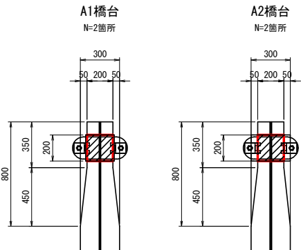
支承交差部詳細図 S=1:20
