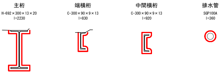
支承交差部詳細図 S=1:20
