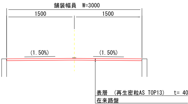
舗装構成（現況） S=1:20
