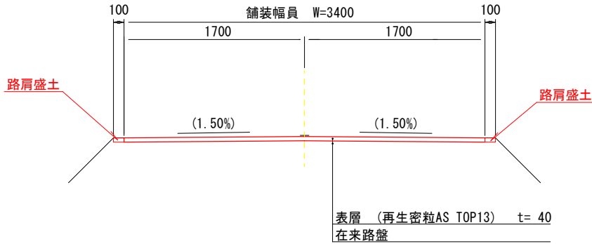
舗装構成（現況） S=1:20
