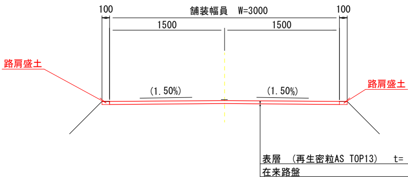
舗装構成（現況） S=1:20
