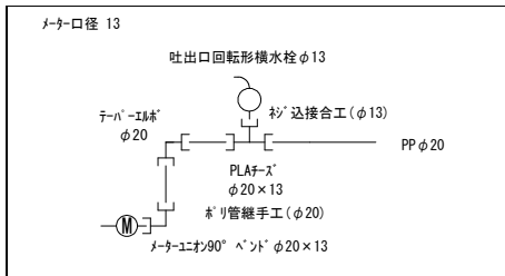
仮設給水管設置工 (メ-タ-φ13)
