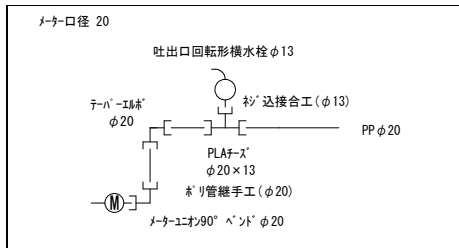
仮設給水管設置工 (メ-タ-φ20)
