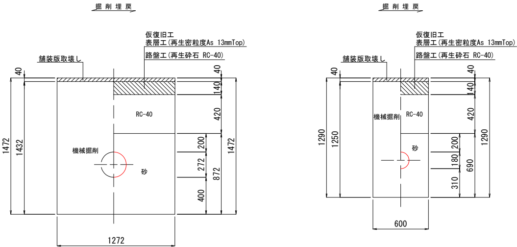
断面図
