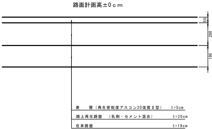
舗装構成 (計画) S=1:10
