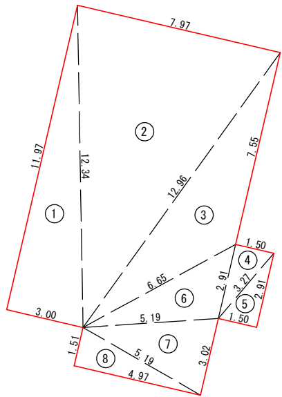
吸出防止材面積求積図
