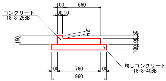
基礎コンクリートD 数量表 10m当り
