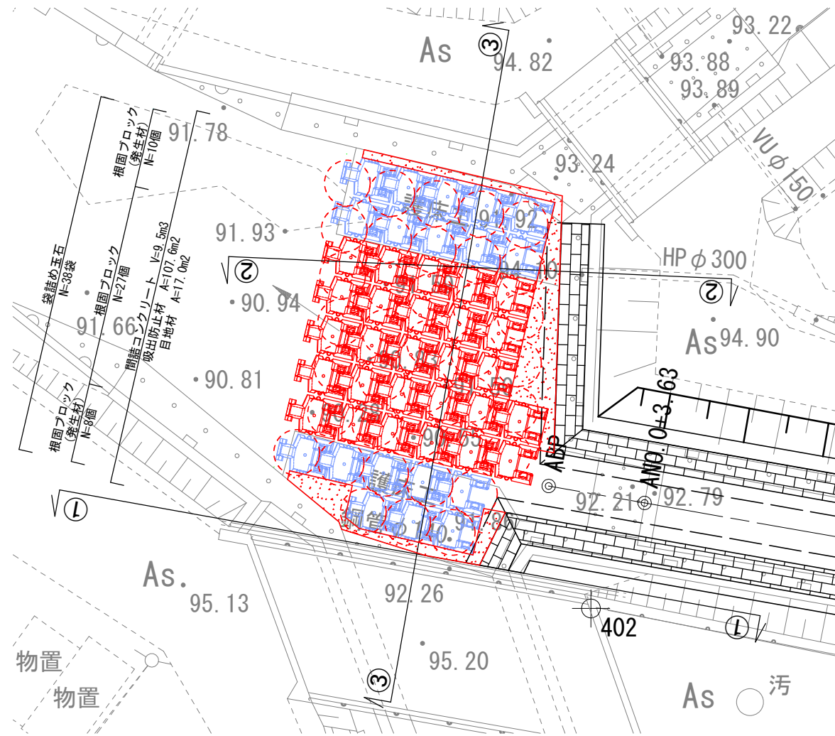
吸出防止材面積求積図
