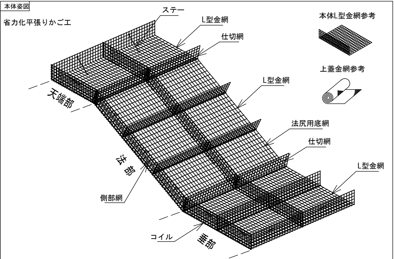
ハイパーマット平張り型H50 省力化平張りかごエ 特記仕様表
