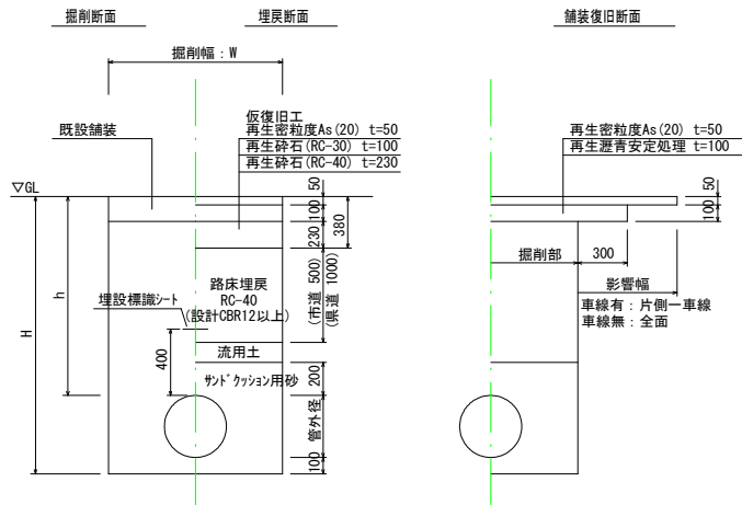
舗装計画交通量250≦T<1000 (N5) 大型車交通量250台以上1000台未満 (B交通)
