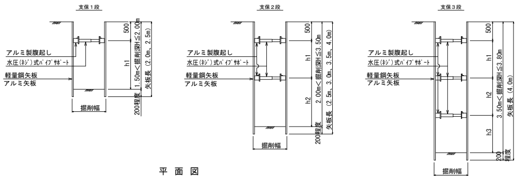
平面図
