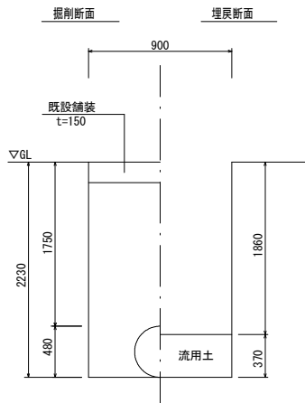
既設管撤去土工断面 (B交通)
