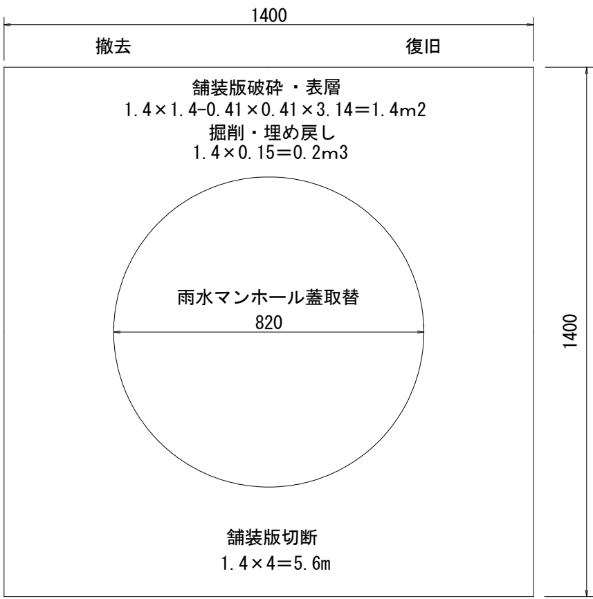
平面図
