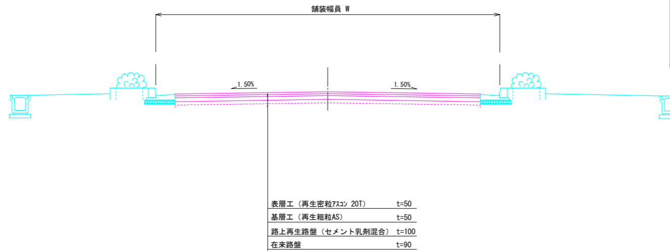
断面図 S=1:50 市道14号線
