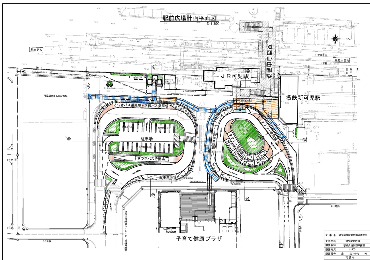
図 可児駅・新可児駅駅前広場計画平面図
