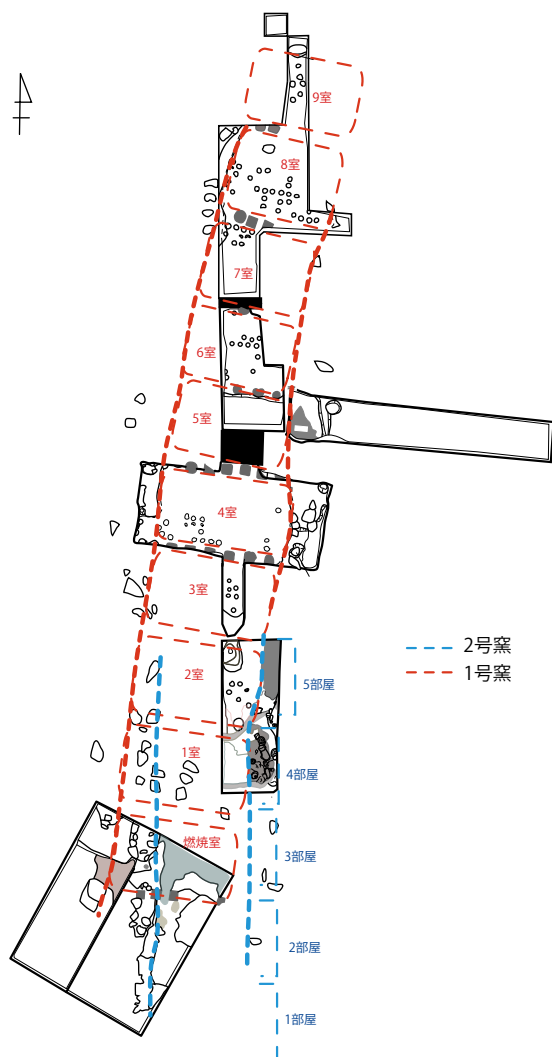
弥七田古窯跡平面図（縮尺は1/170）
